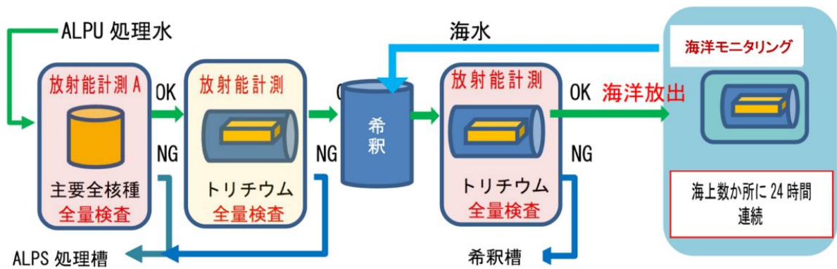
図 1 トリチウム連続計測システム概要
