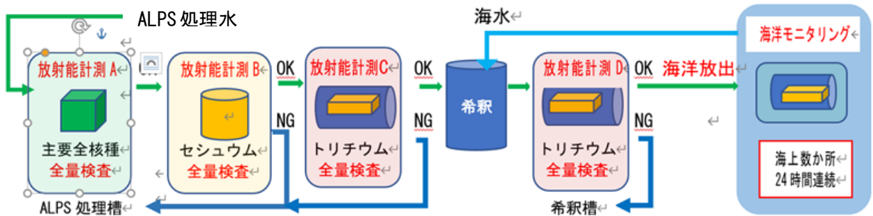
図1 トリチウム連続計測システム概要
